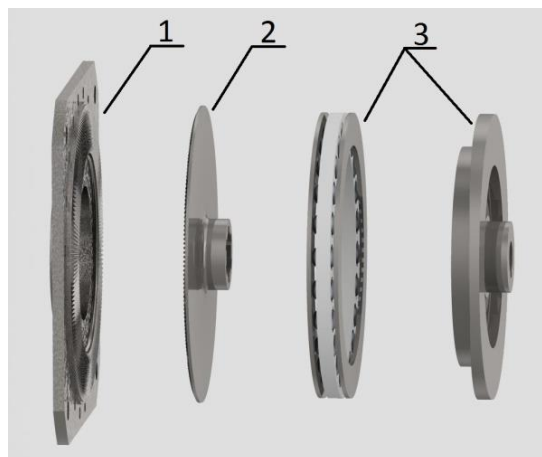
1. ábra. A síkkerekes hullámhajtómű alapelemei: merev kerék (1), hullámkerék (2), rugalmas csapágy és bütökös hullámgenerátor (3) (Kardos és Krisch, 2015)
