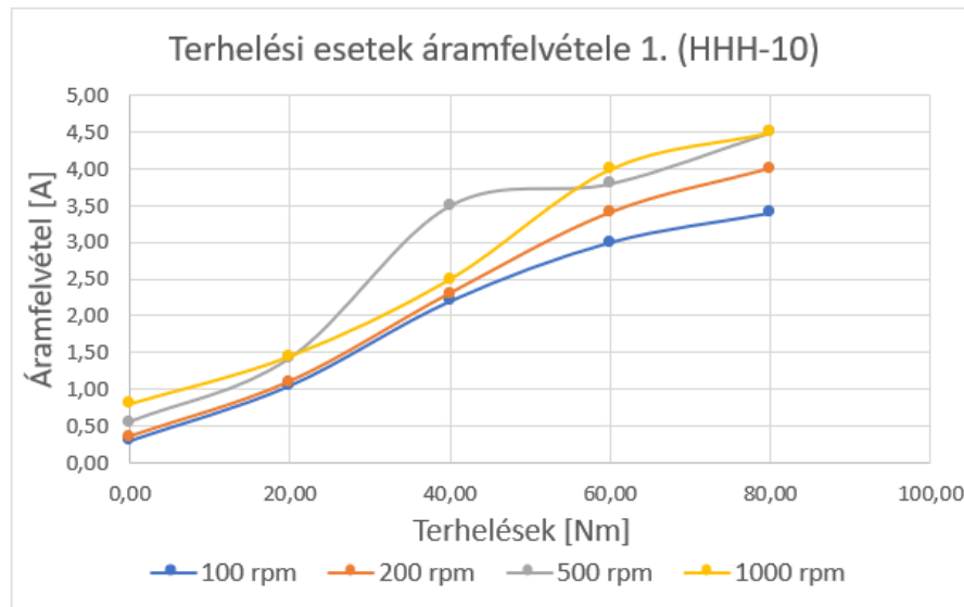
6. ábra. HHH-10 hajtásrendszer áramfelvétele
