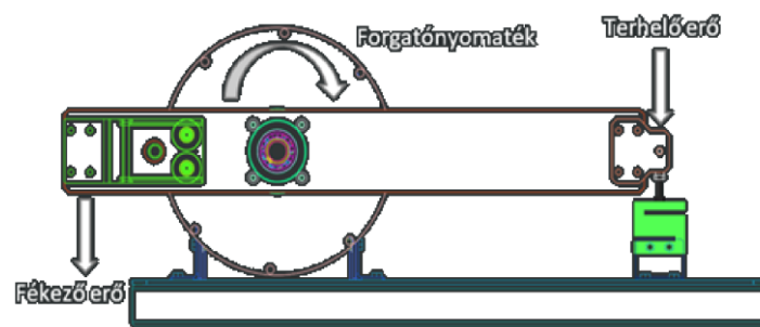
3. ábra. Hajtásrendszer tesztelő próbapad
