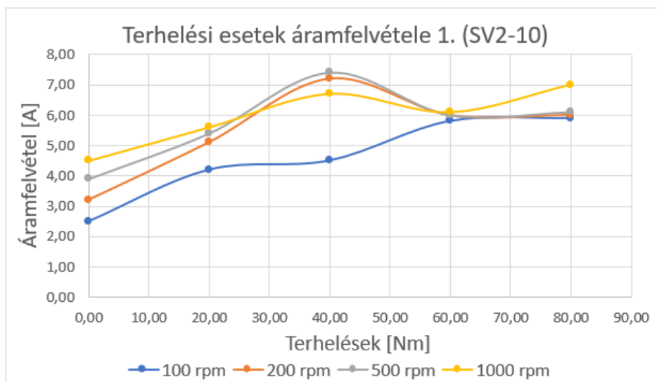
5. ábra. SV2-10 hajtásrendszer áramfelvétele
