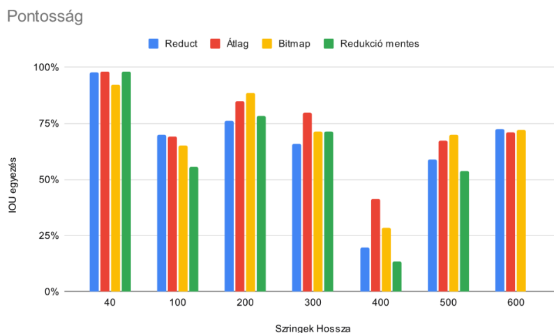
Figure 3. Pontosság
