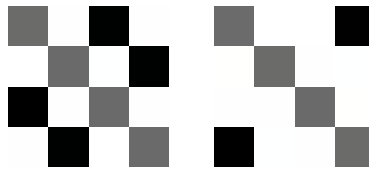
Figure 1. Egyezésmátrix képként
