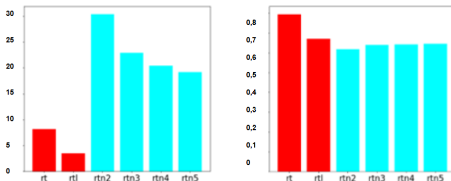
3. ábra. Wine adathalmaz futási ideje, valamint hiba mértéke
