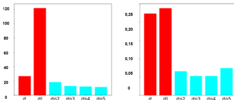
1. ábra. Blob adathalmaz futási ideje, valamint a hiba mértéke
