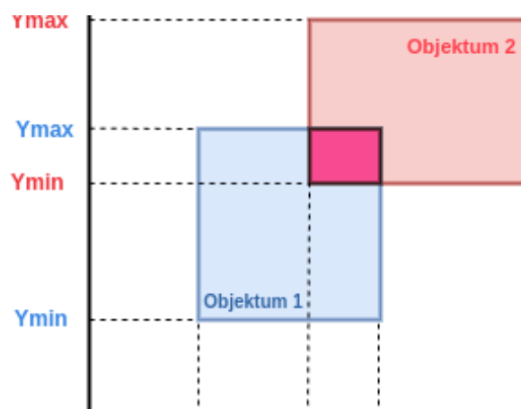
4. ábra. AABB alapú ütközés
